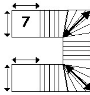
3 escaliers droit, 2 courbe
